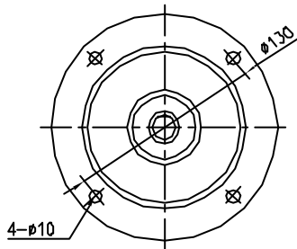
VIEW A-A
